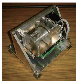
親子衛星実験装置「テザー機構ダイナミックシュミレーター」
