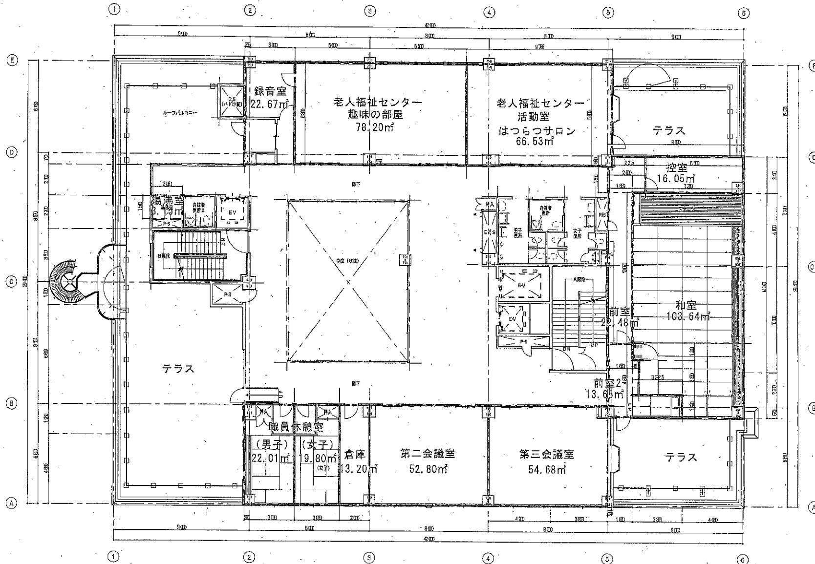
田無総合福祉センター4階現況図
