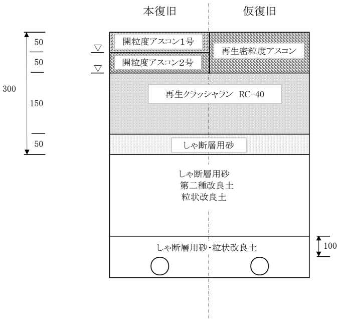
□ 透水性アスファルト舗装 30型
