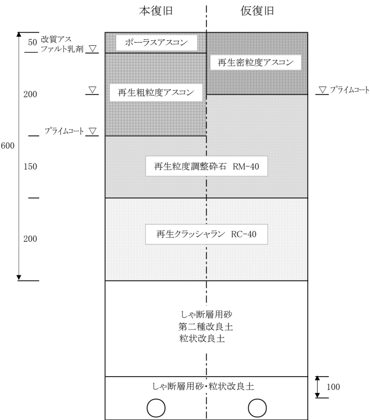
□ 排水性アスファルト舗装 60型
