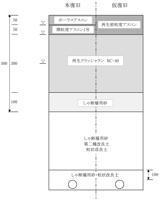
□ 排水性アスファルト舗装 60型
