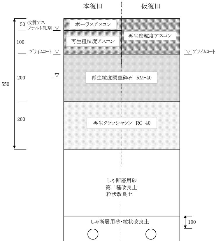
□ 排水性アスファルト舗装 55型
