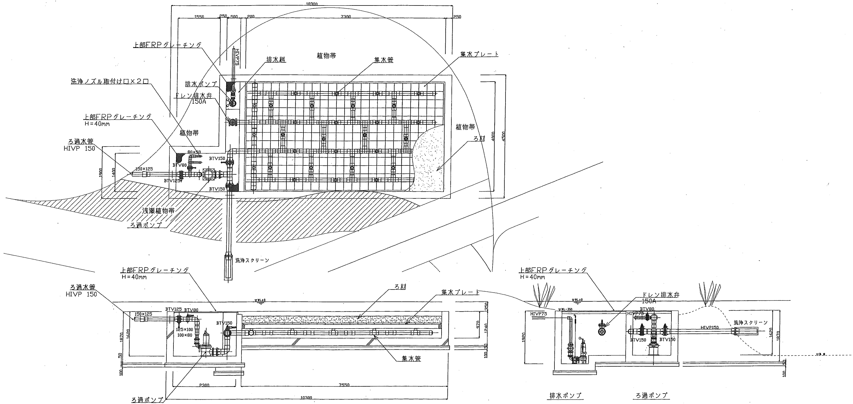
生物ろ過装置詳細図
