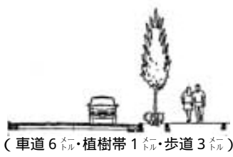
道路標準断面図 (車道と歩道の間に植樹)
