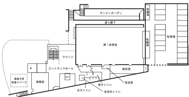
1階平面図
