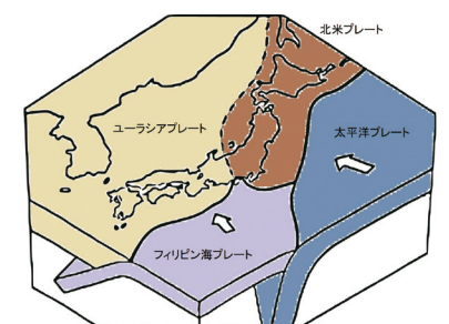
▲日本列島付近のプレートの分布
