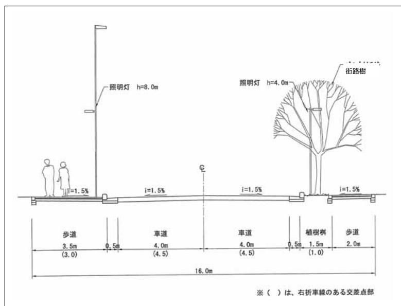
都市計画道路 西 3・4・21 号の標準断面図
