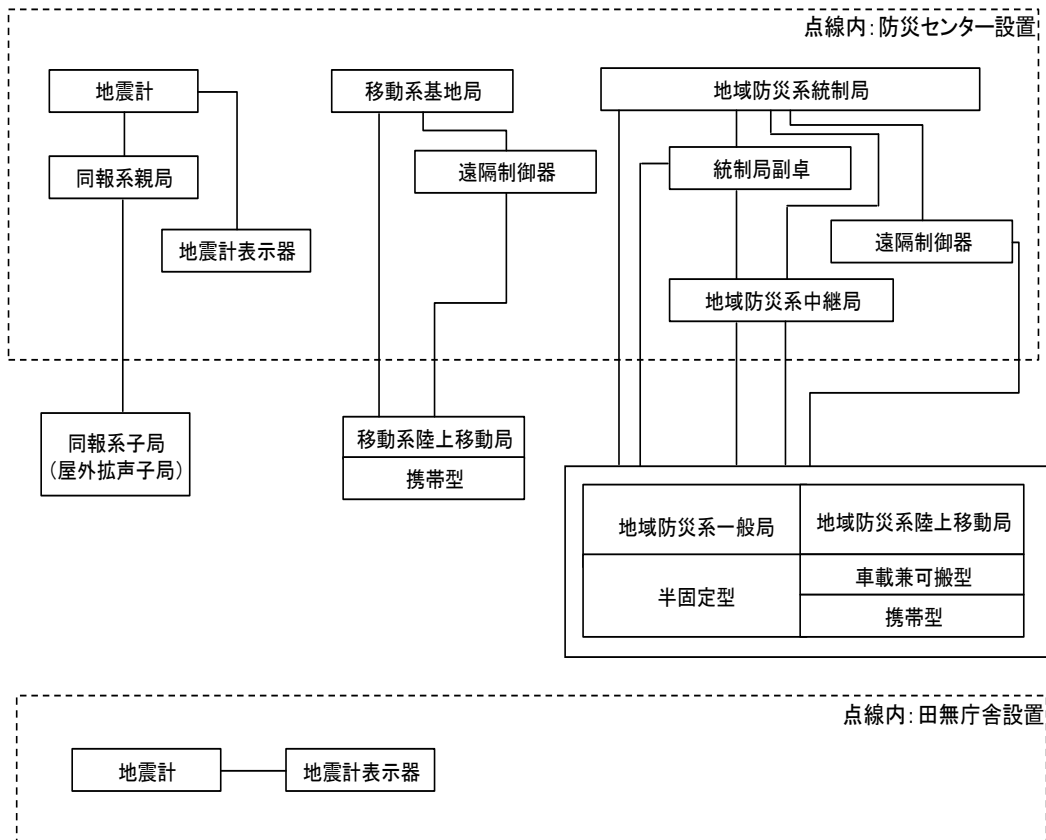
【市防災行政用無線局回線構成図】
