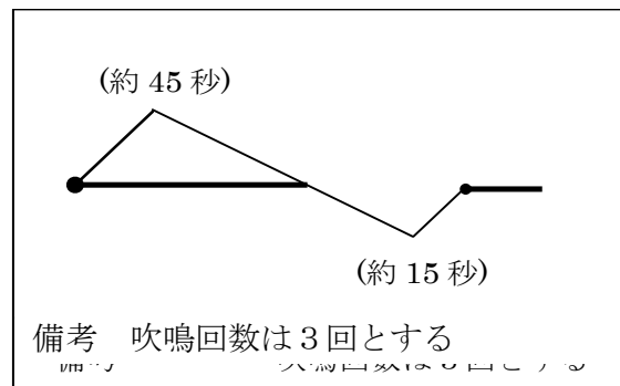
【防災信号（サイレン）の吹鳴パターン】
