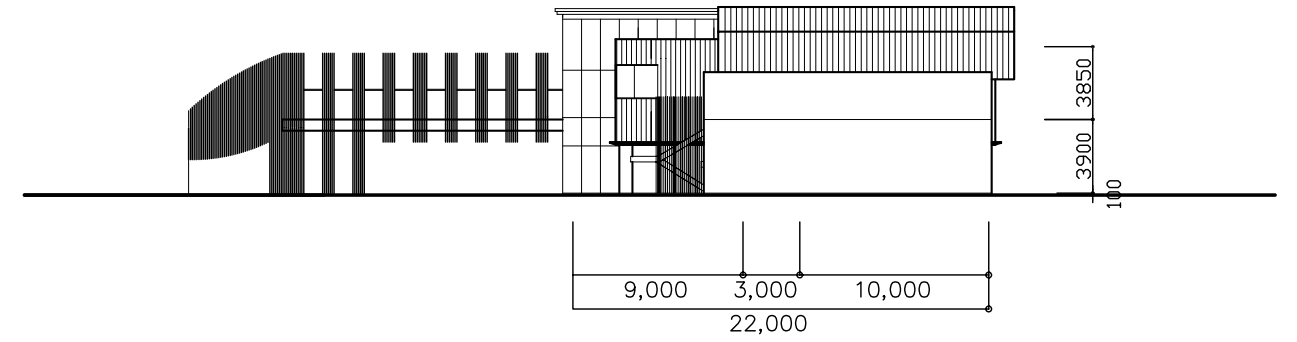
北立面図
