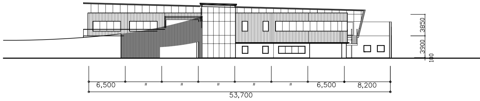
西立面図
