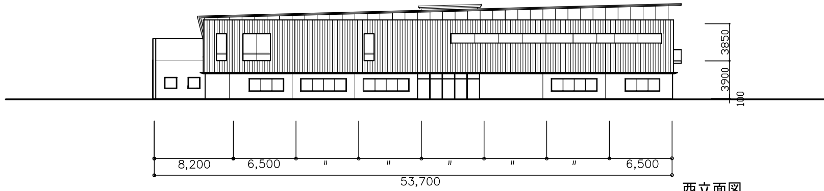
西立面図
