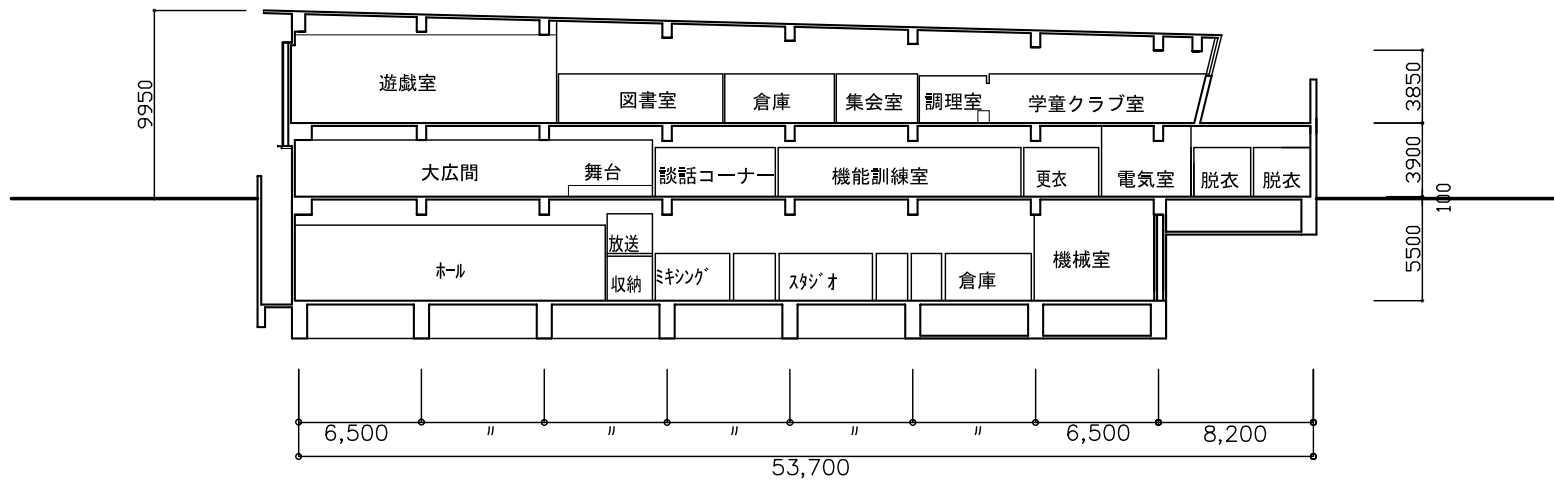
南北断面図
