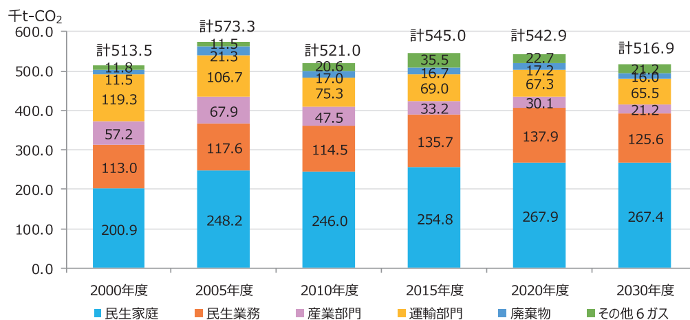
図 温室効果ガス排出量の将来予測
