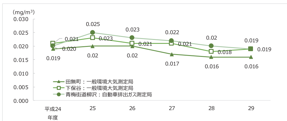
図 大気中の浮遊粒子状物質（SPM）の測定結果（年平均値）
