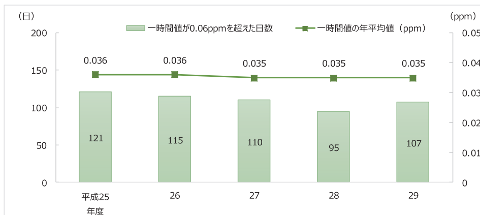
図 大気中の光化学オキシダントの測定結果（日数、年平均値）
