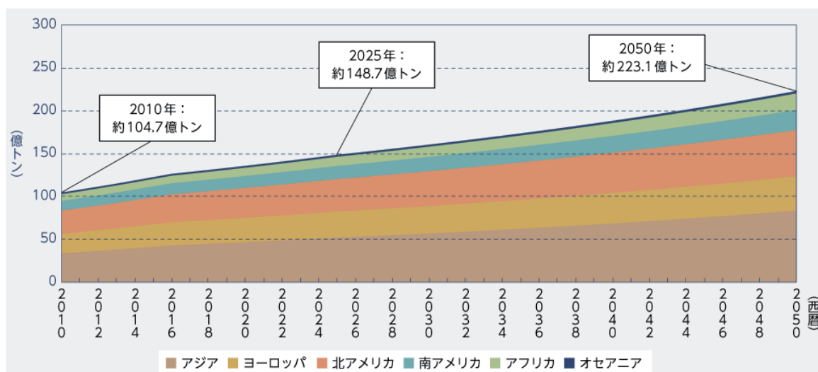
図 世界の廃棄物発生量の将来予測
