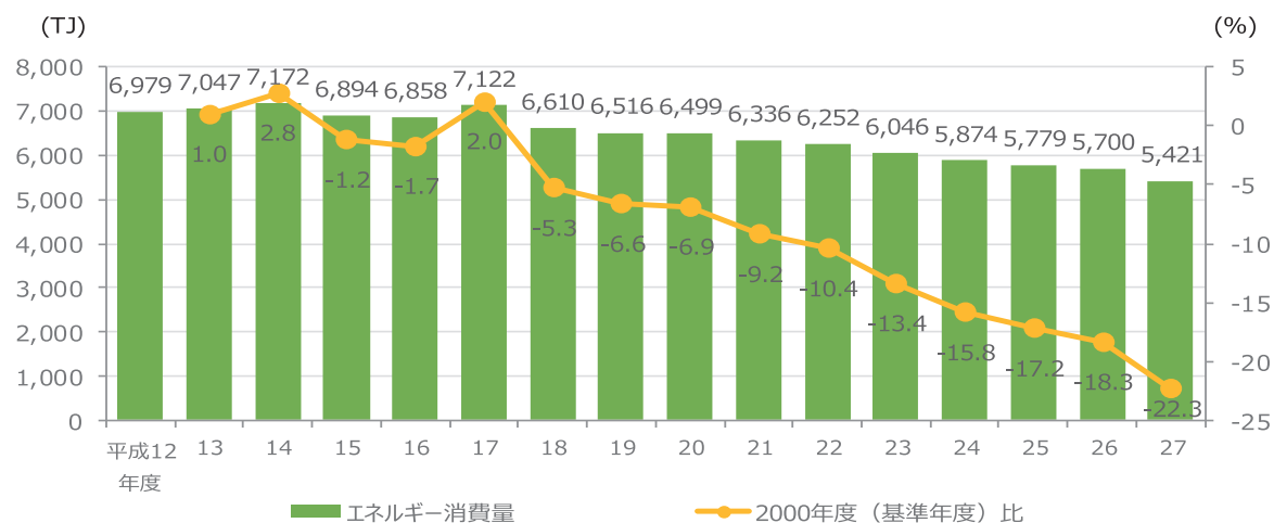
図 エネルギー消費量の推移
