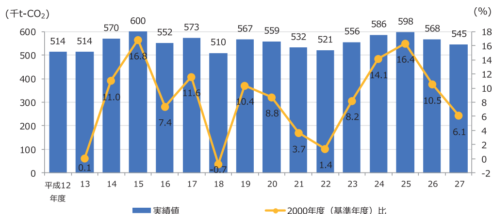
図 本市の温室効果ガス排出量の推移
