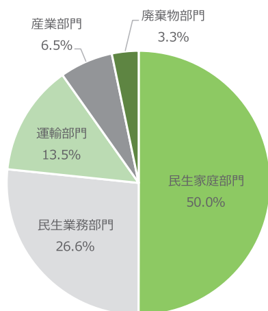
図 部門別二酸化炭素排出量 (平成 27 年度)
