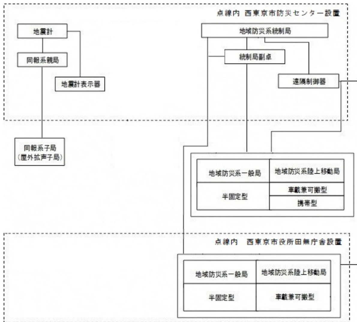
西東京市防災行政用無線局回線構成図
